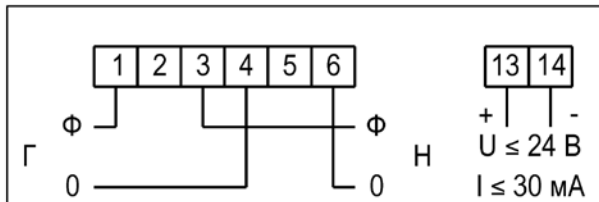
Рисунок В.2 – Схема включения счетчиков CE 102 тип корпуса S6, исполнения «О»
