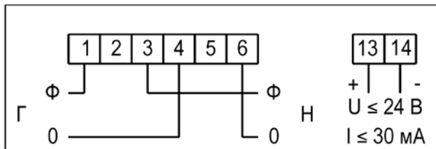
Рисунок В.4 – Схема включения счетчиков CE 102 тип корпуса R5, исполнения «О»
